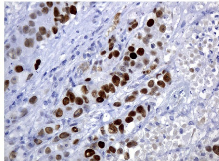
Lung Adenocarcinoma
